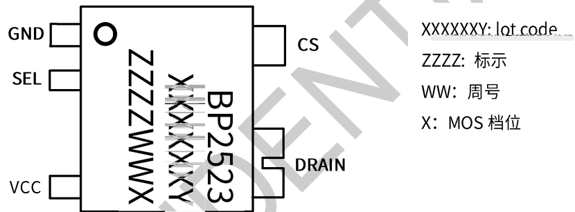
图 2 管脚封装图
